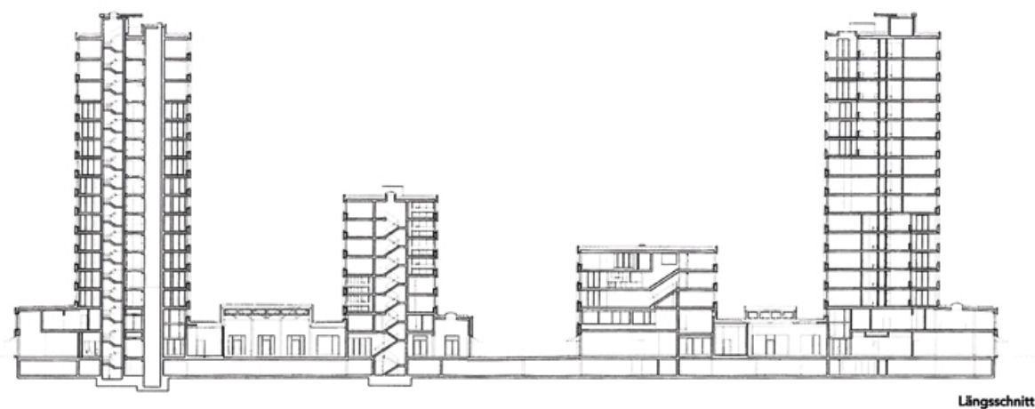
Längsschnitt
