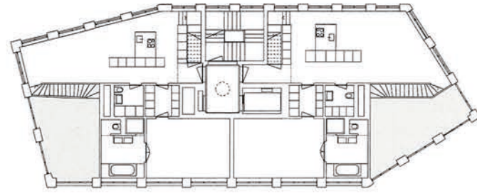
Pianta livello 10
