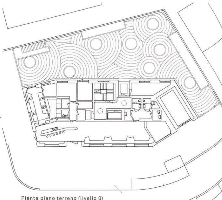
Pianta piano terreno (livello 0)
