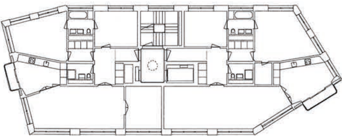
Pianta livelli 1-4
